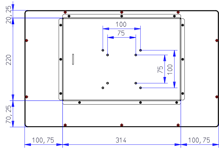
Rückansicht
