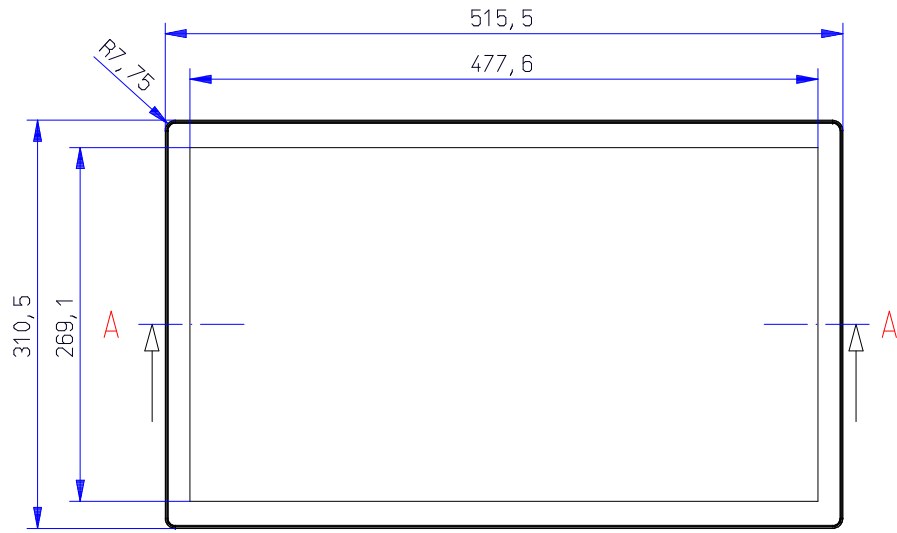
Frontansicht
